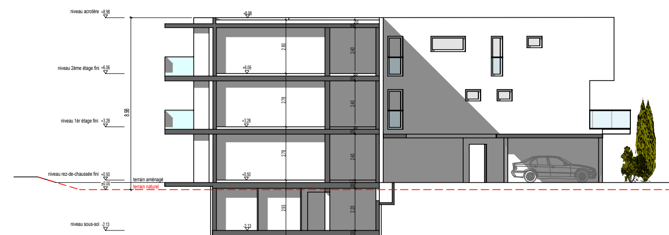
coupe AA
